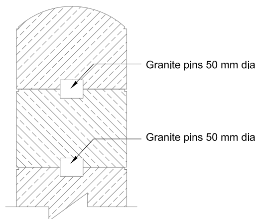
Detail-E
