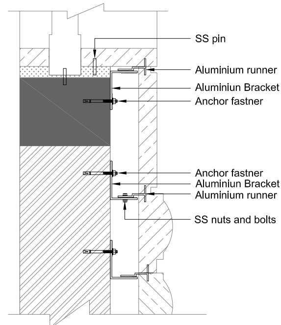
Detail-B
